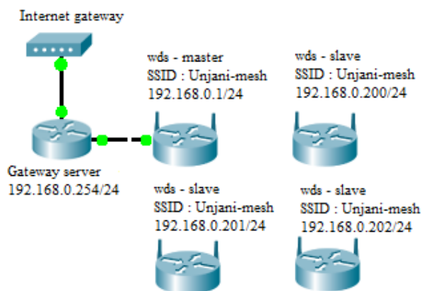
Gambar 5. Topologi jaringan WDS
