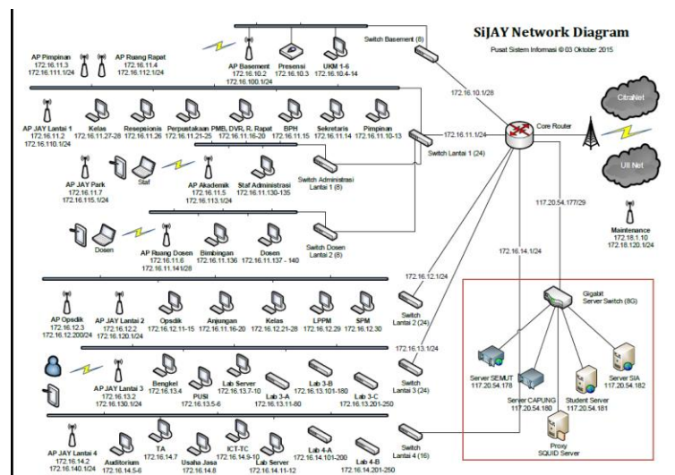
Gambar 3. Kondisi Topologi yang Berjalan
