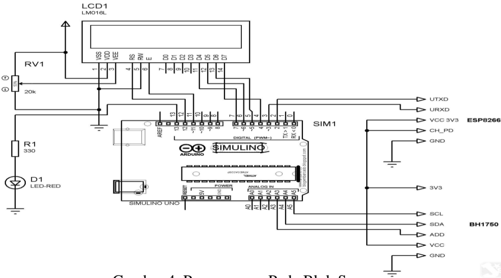
Gambar 4. Perancangan Pada Blok Sensor
