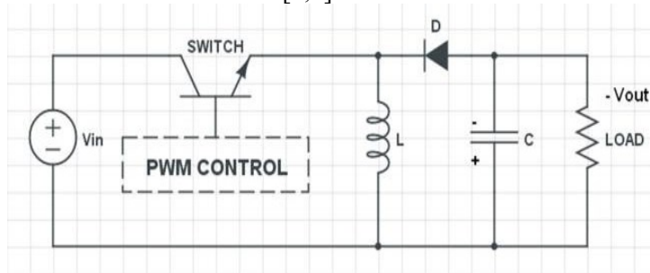
Gambar 5. Rangkaian Ekivalen Buck Boost Converter
