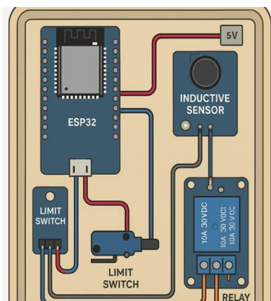
Gambar7. Desain rangkaian pcb
