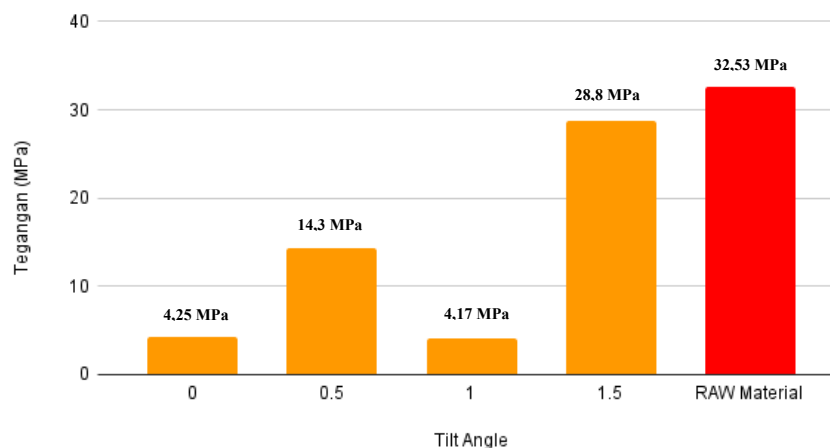
Gambar 14. Chart Hasil Pengujian Bending
