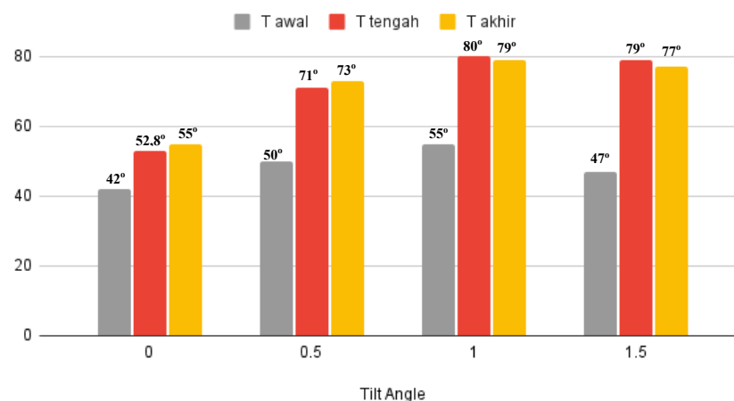
Gambar 8. Chart Suhu awal, tengah, dan akhir proses FSW
