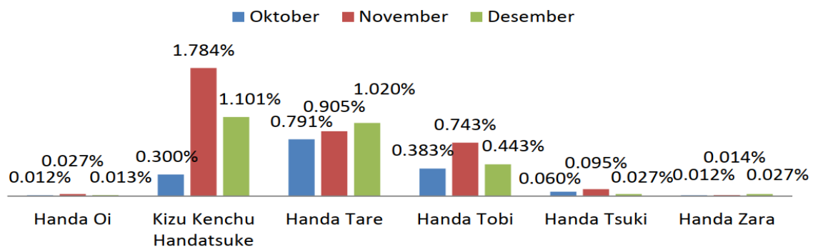
Gambar 4. Persentase Defect pada Body Flute
