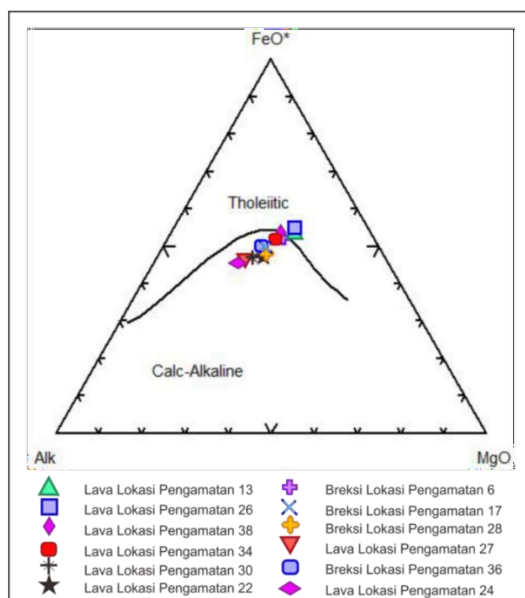
Gambar 6. Hasil plot geokimia pada diagram AFM (Alkali, Feroksida, dan Magnesia), menunjukkan tipe calc-alkaline (10 sampel), dan tholeiitic (2 sampel).
