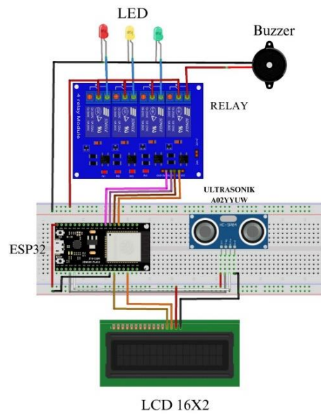
Gambar 10. Rangkaian Skematik Sistem Pendeteksi Banjir
