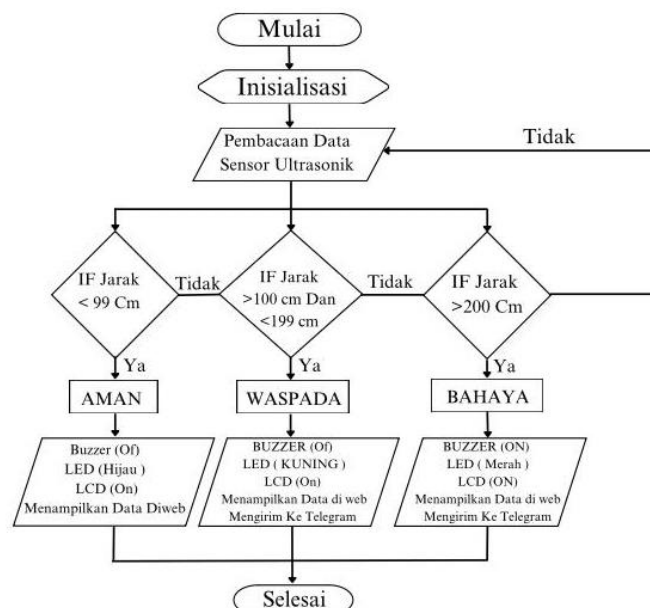
Gambar 1. Diagram alir kerja rangkaian
