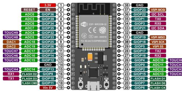
Gambar 4. ESP 32
