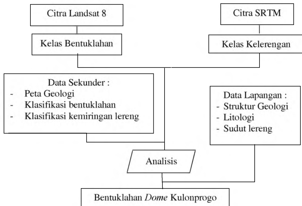
Gambar 2. Diagram Alir Tahapan Penelitian
