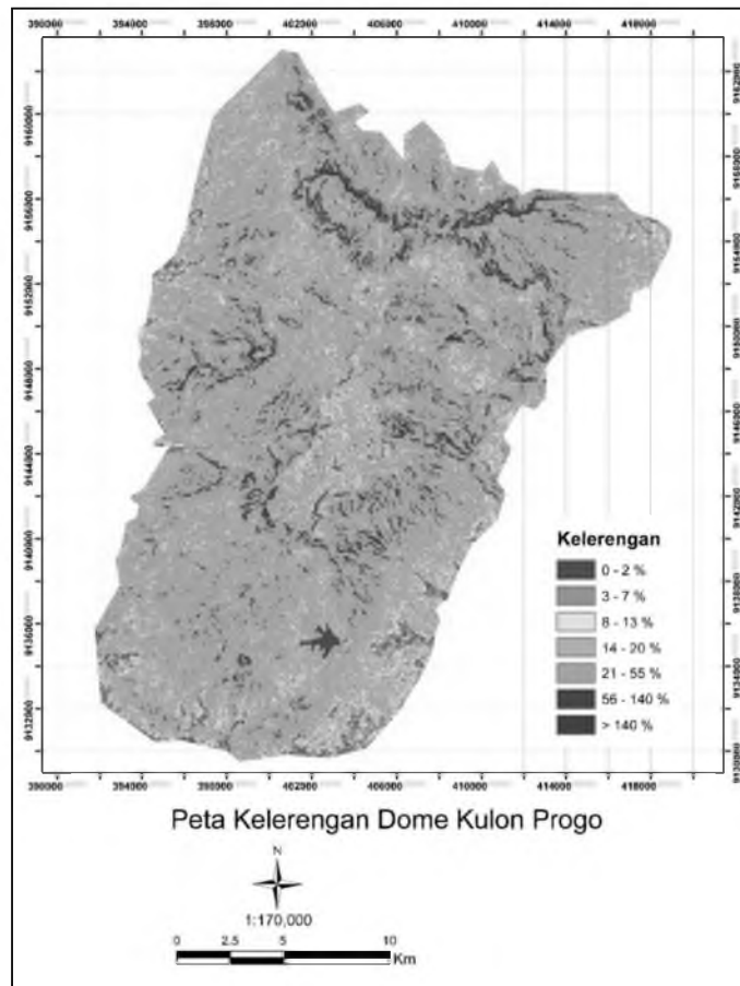
Gambar 3. Hasil kelas lereng Dome Kulonprogo
