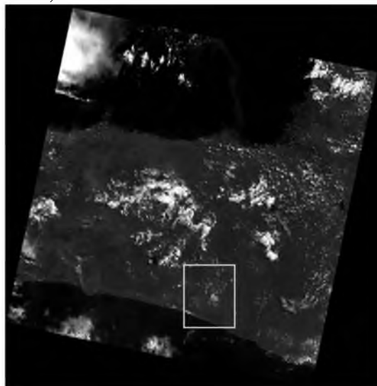
Gambar 1. Lokasi Penelitian di Dome Kulonprogo
