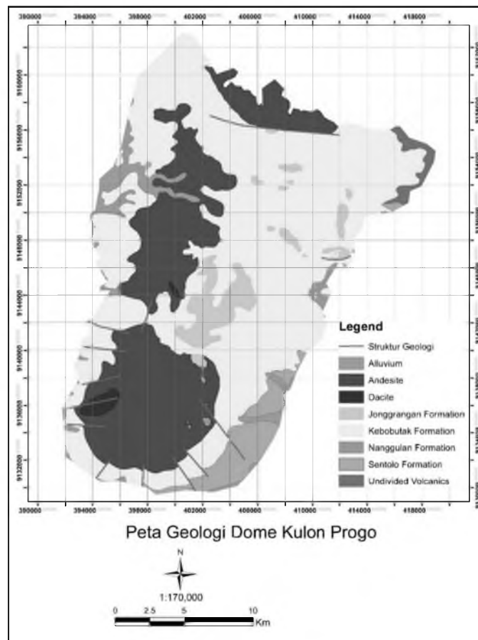
Gambar 4. Peta Geologi Dome Kulonprogo
