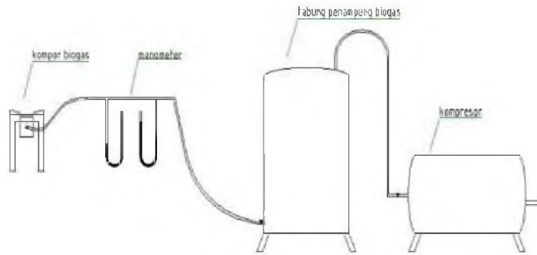
Gambar 4. Instalasi percobaan
