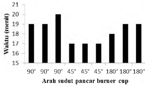
Gambar 11. Grafik perbandingan konsumsi biogas untuk mendidihkan air masing-masing percobaan
