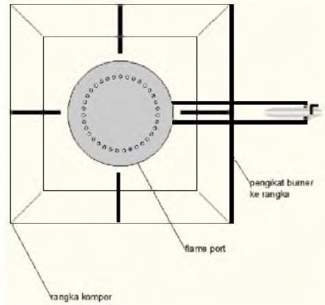
Gambar 5. Tampak atas desain kompor hasil perhitungan.
