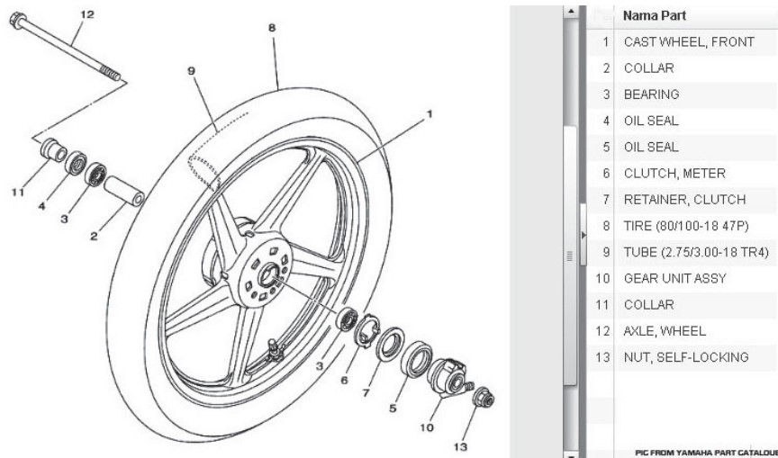
Gambar 1. Rangkaian komponen pada poros roda
