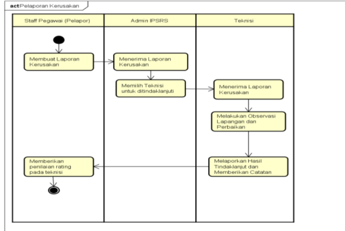
Gambar 3. Activity diagram pelaporan kerusakan
