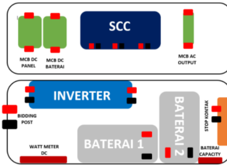
Gambar 2. Desain dari komponen generator portable tenaga surya
